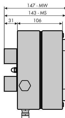
Version avec IHM eNodTouch MS/MW - Version with HMI eNodTouch MS/MW
