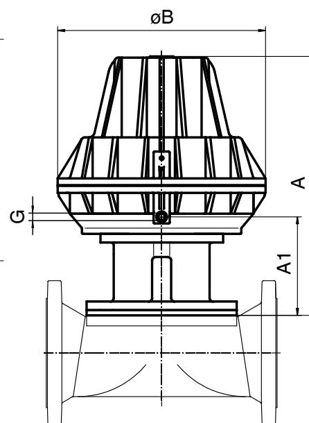
Actuator size 4
